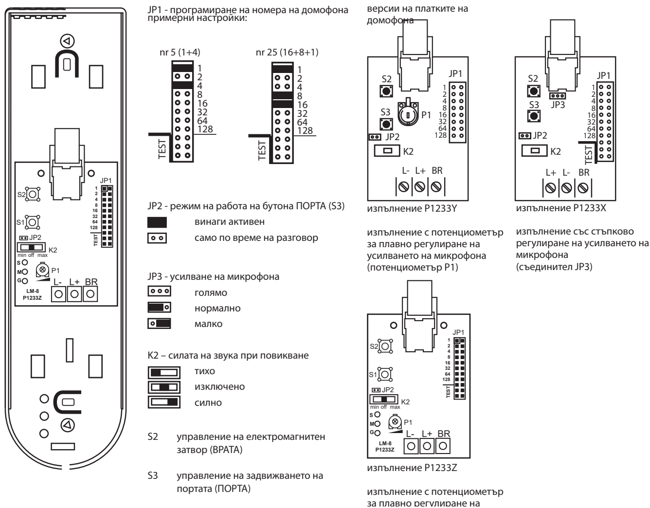
Фиг. 5. Клеми, конфигурационни джобри и регулаторни елементи на печатната платка на унифона.
