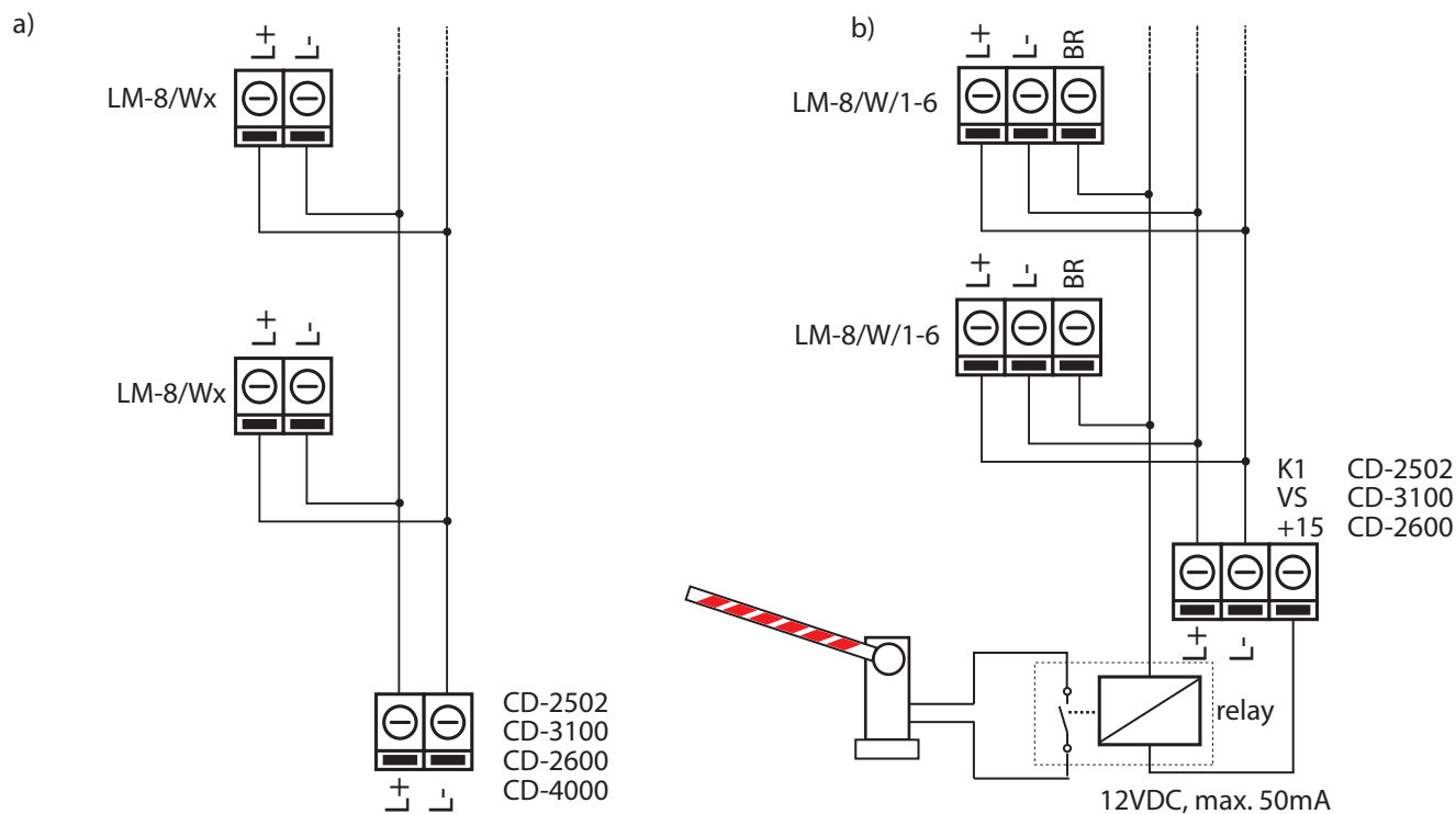
Фиг. 3. Свързване на унифона към домофонната система.
