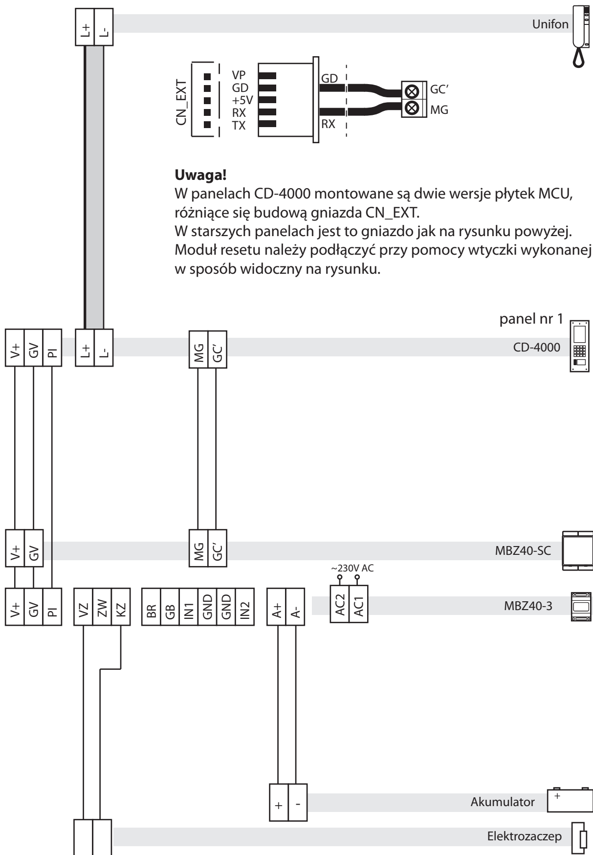
Rys. 2. Schemat podłączenia modułu MBZ40-SC.
