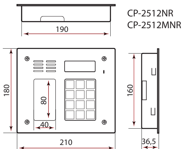
Rys. 8 Wymiary z listą lokatorów, INOX
