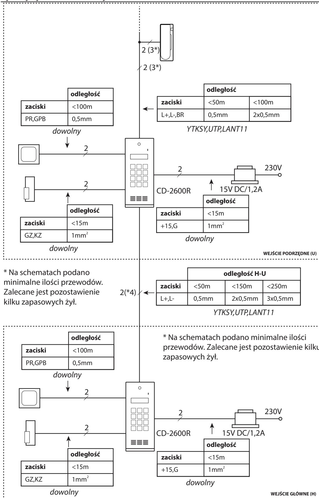
Rys. 11.2. System wielowejsciowy. Liczba przewodów i dopuszczalne odległości.
