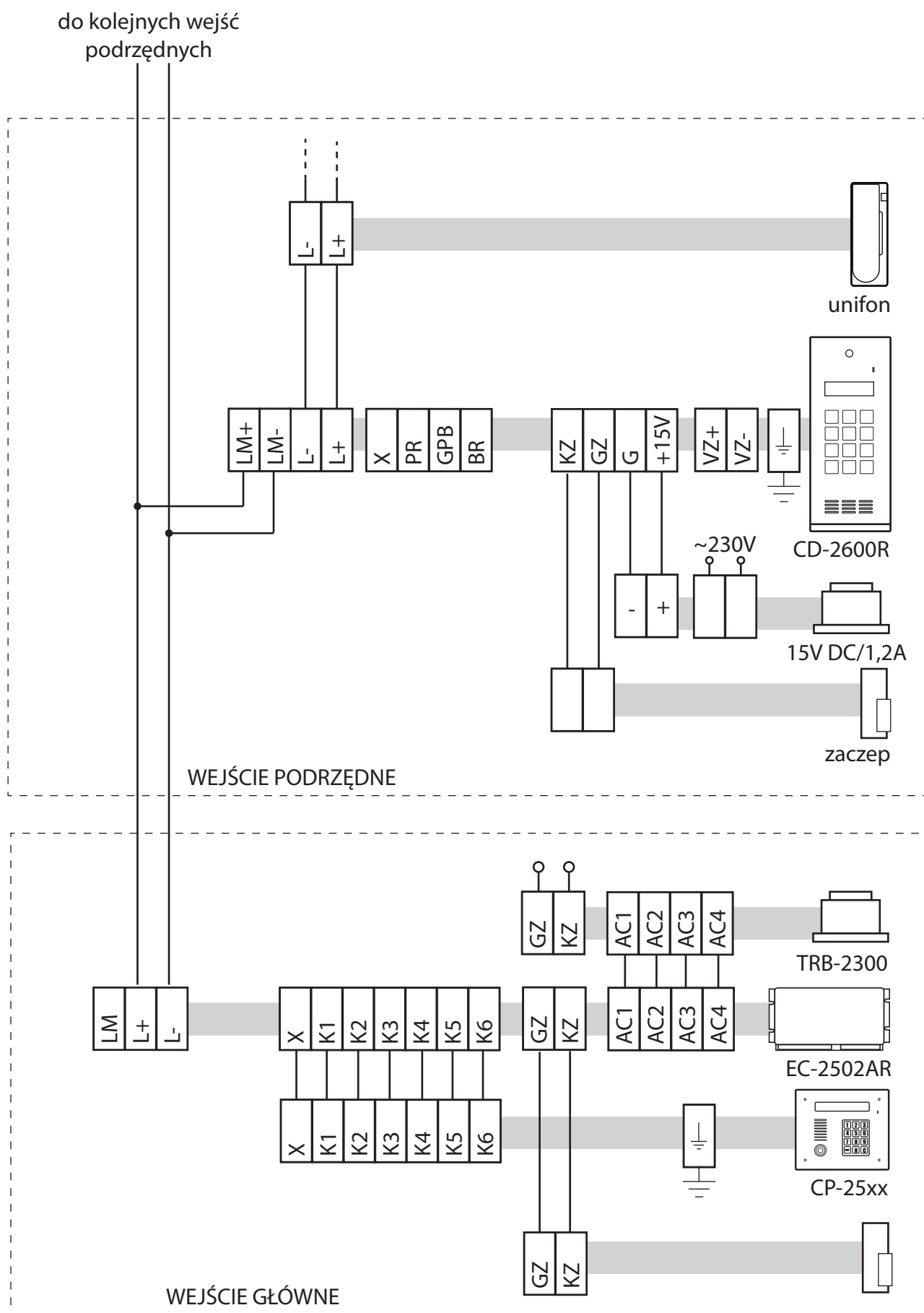
Rys. 11.7. Współpraca z CD-2502/3000. CD-2600 jako wejście podrzędne.
