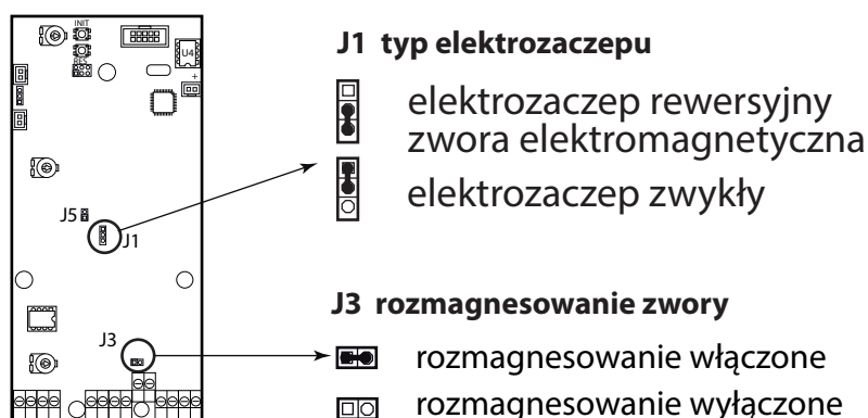
Rys. 5.1. Konfiguracje zworek J1 i J3 na płycie w panelu zewnętrznym.
