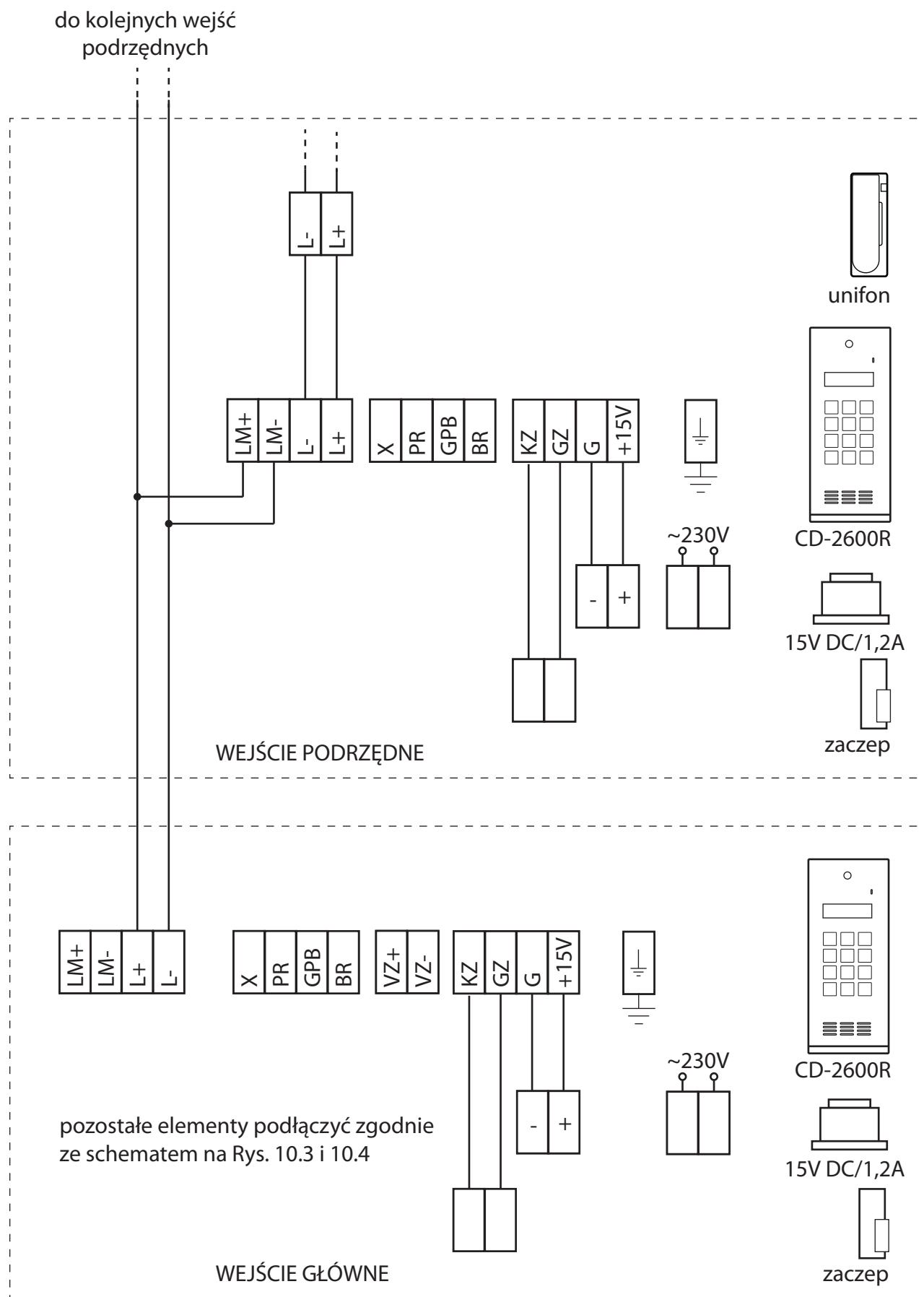
Rys. 11.5. System z wejściem głównym.
