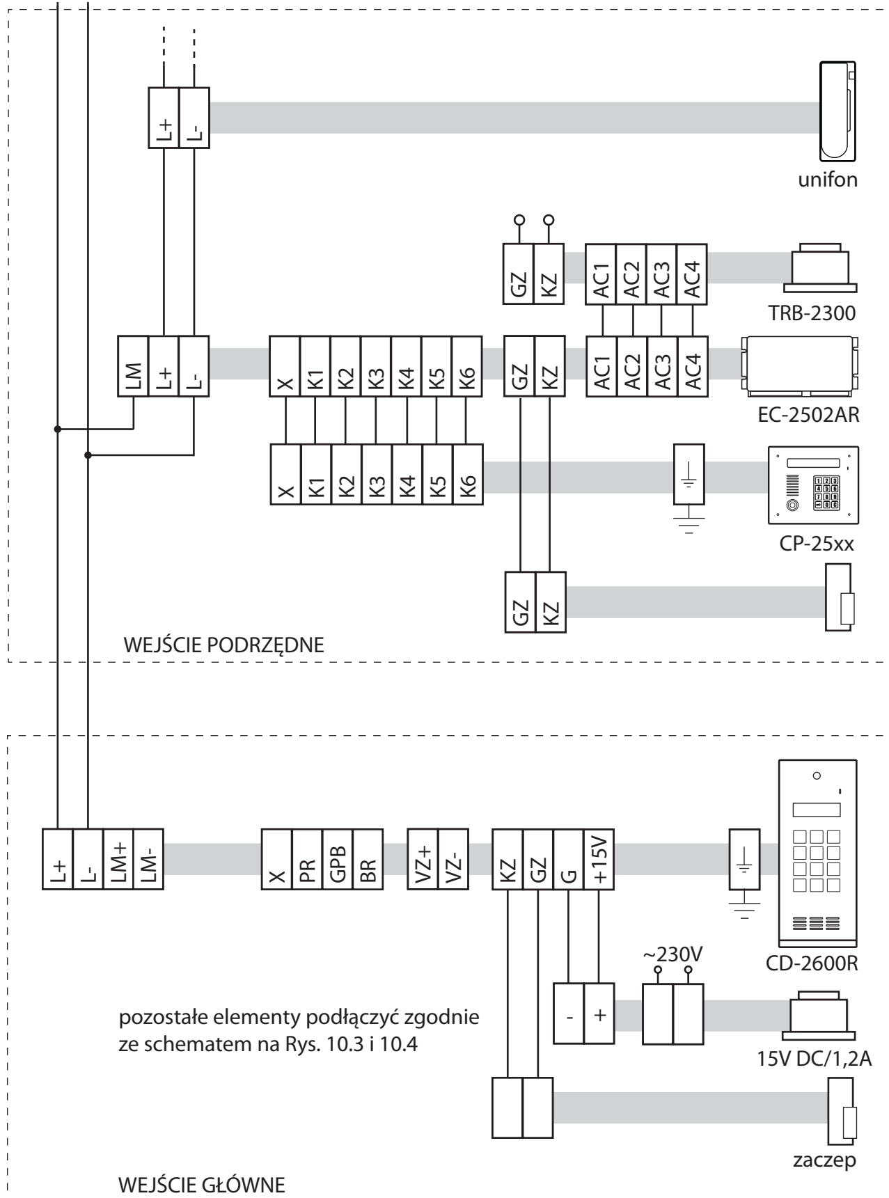
Rys. 11.6. Współpraca z CD-2502/3000. CD-2600 jako wejście główne.
