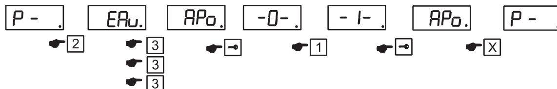
Rys. 6.4. Procedura P2 na przykładzie zmiany wartości parametru APo. Domyślna wartość 0 została zmieniona na 1.
