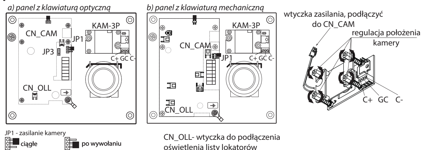
Rys. 6.7. Moduł kamery i panel zewnętrzny CP-25xx.
