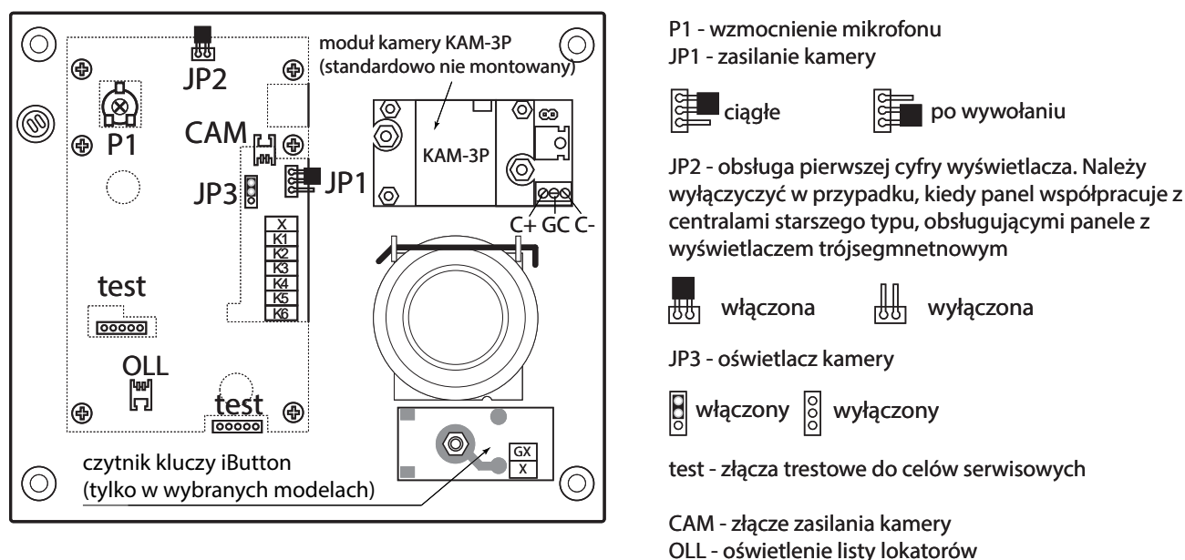
Rys. 13.3. Zaciski w panelach zewnętrznych CP-25XXxx.
