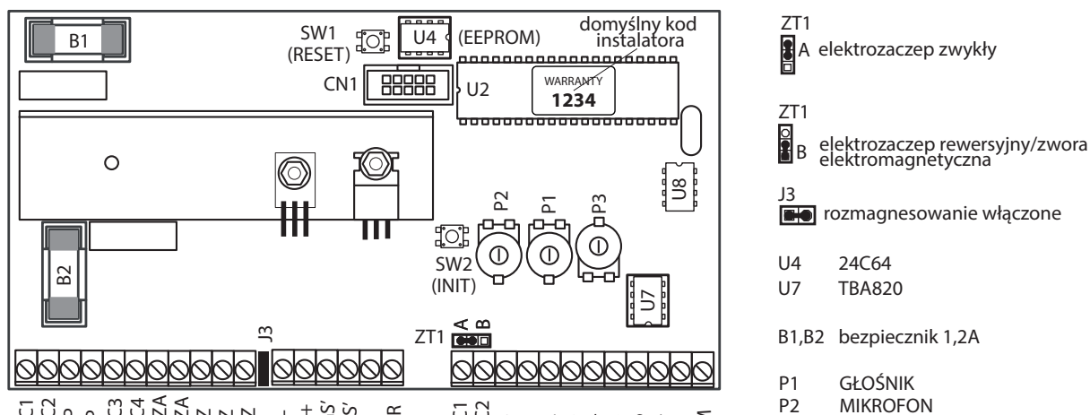
Rys. 13.1. Zaciski centrali domofonowej EC-2502.
