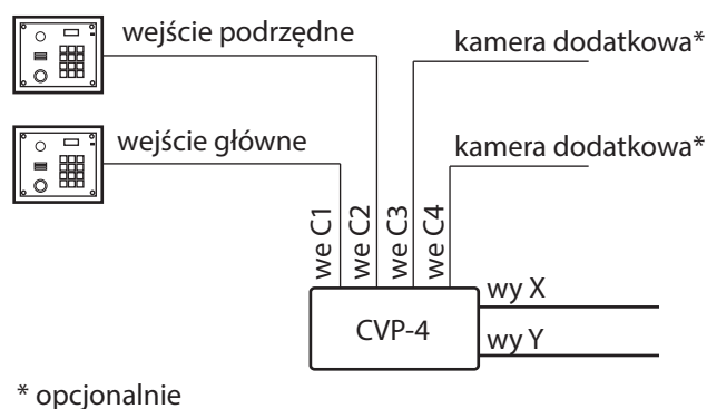
Rys. 6.8. Podłączenie sygnałów z kamer w panelach zewnętrznych do przełącznika CVP-4.
