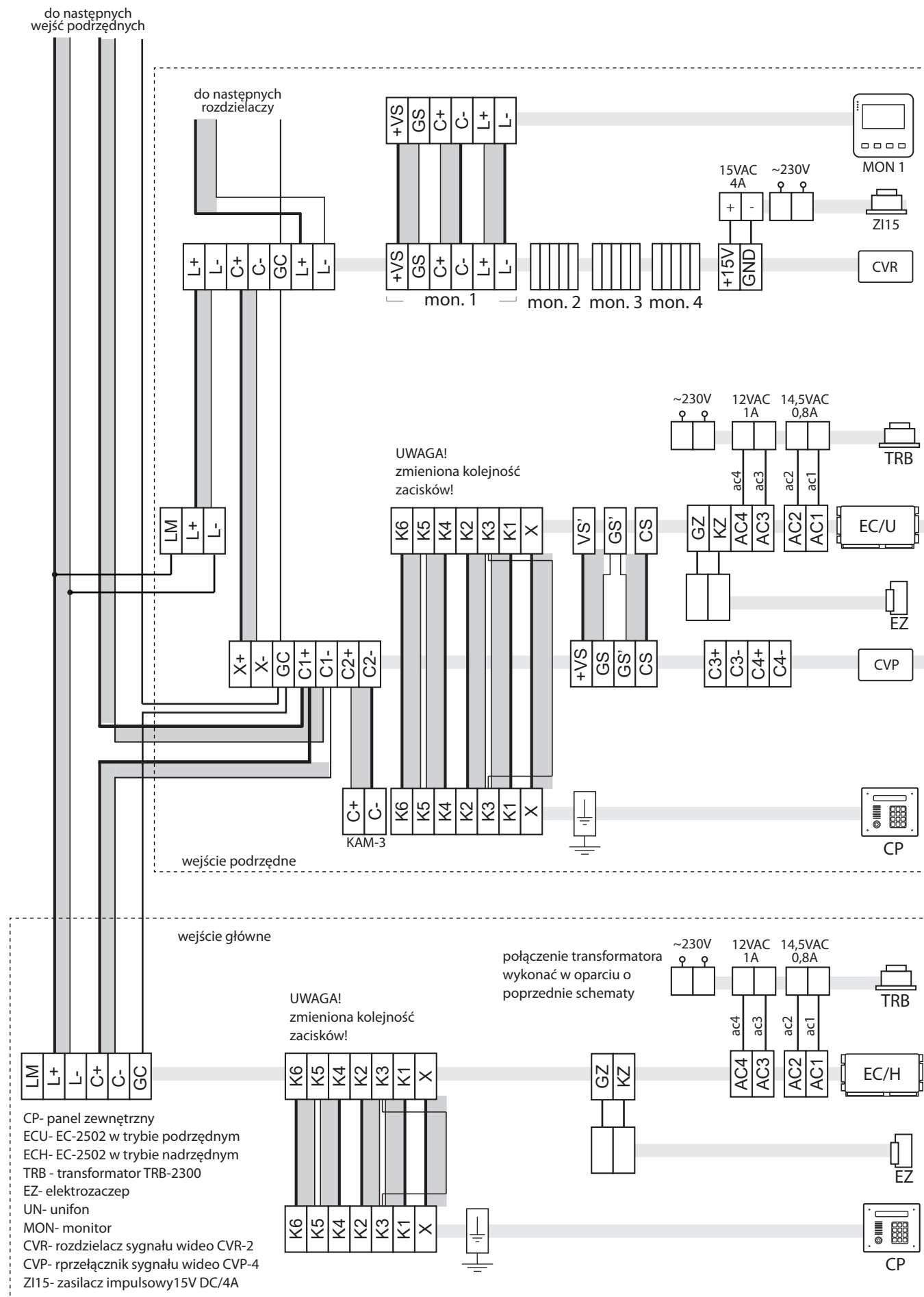
Rys. 14.8. System video z wejściem głównym.
