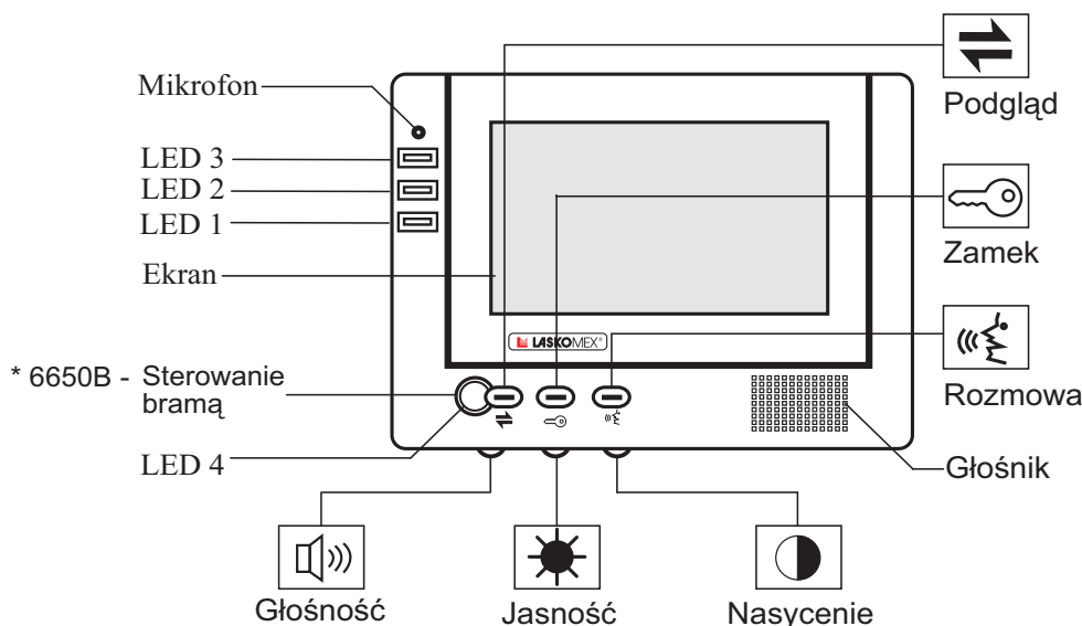
Rys. 1 Widok monitora MVC-6650/6650B
