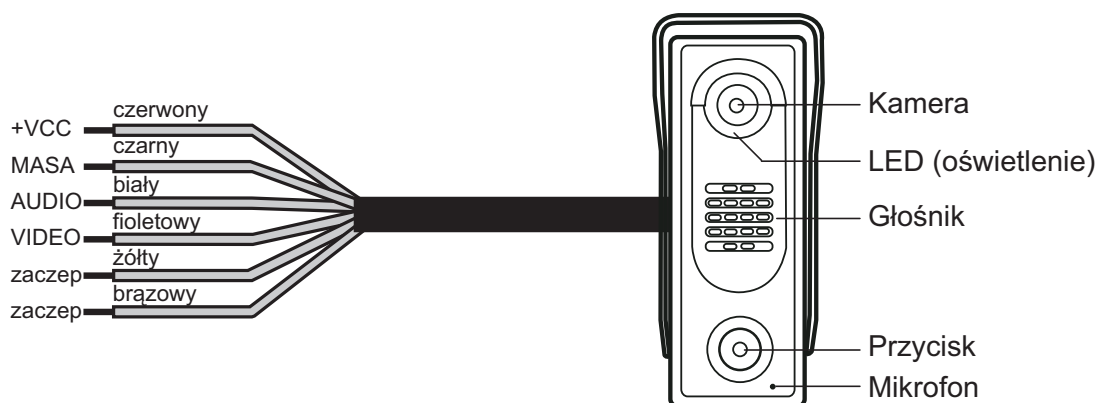
Rys 4. Panel piętrowy BVC-6501
