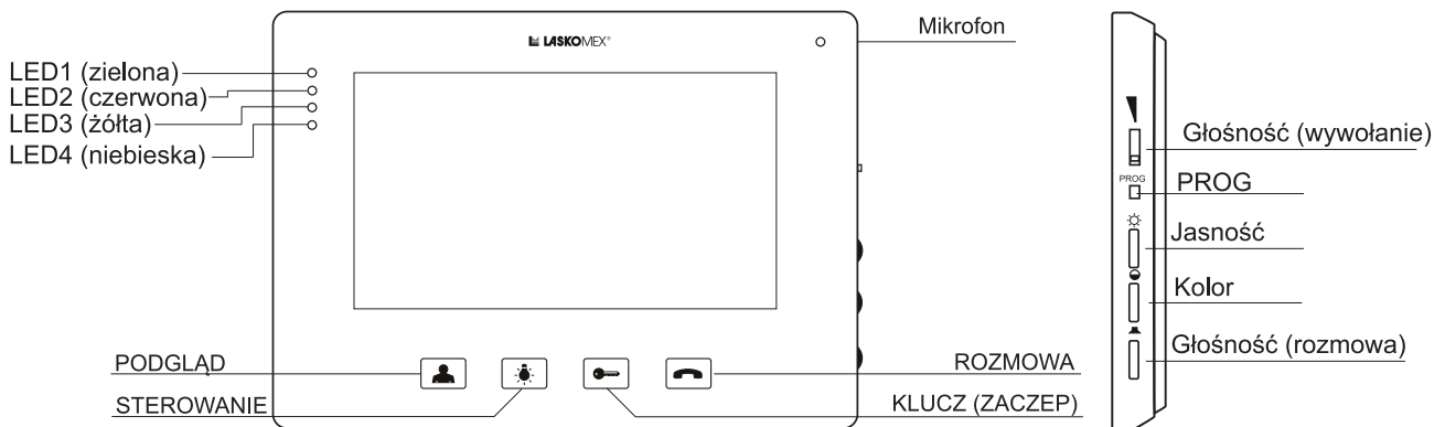
Rys. 1. Monitor MVC-8150
