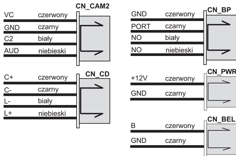
Rys. 5. Opis wtyczek podłączeniowych monitora
