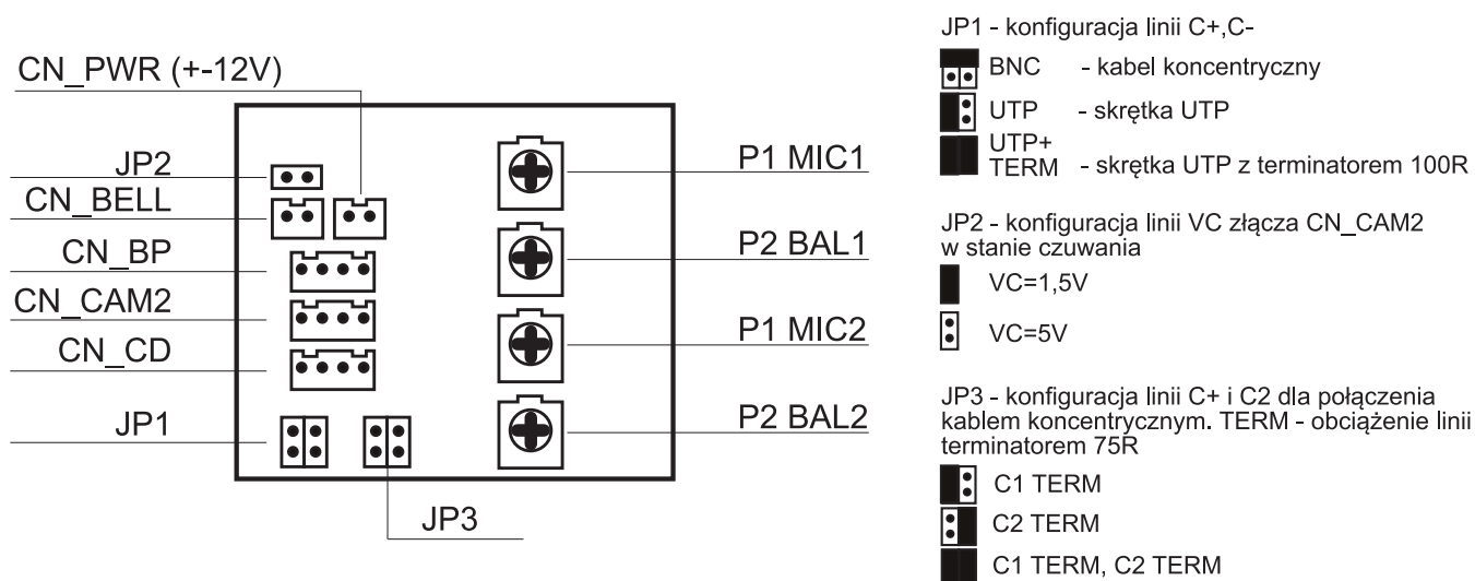
Rys. 6. Opis gniazd podłączeniowych monitora. Elementy regulacyjne i zworki konfiguracyjne
