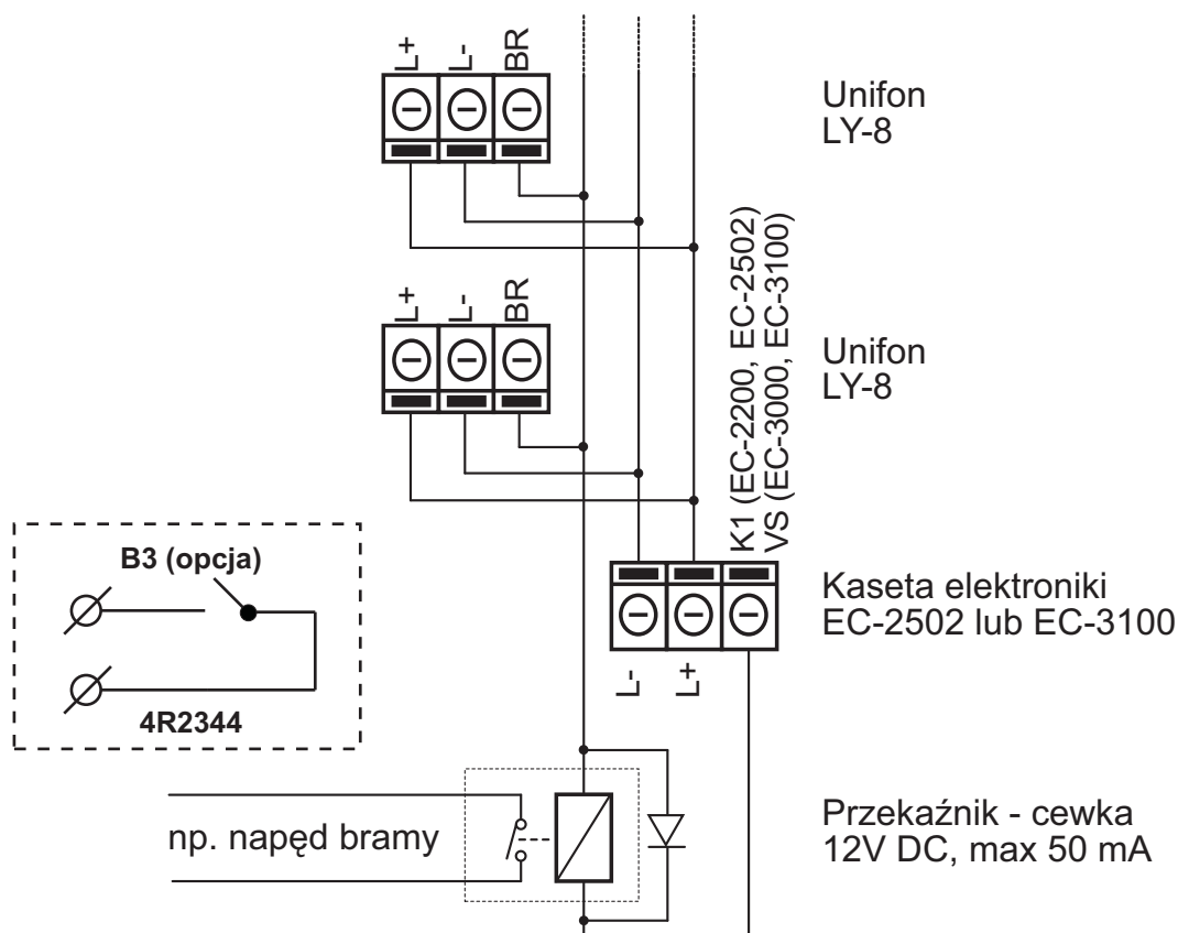
Rysunek 1: Schemat podłączenia urządzenia dodatkowego
