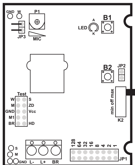
Rys. 3. a) Elementy unifonu LY-8, b) płytki PCB unifonu
