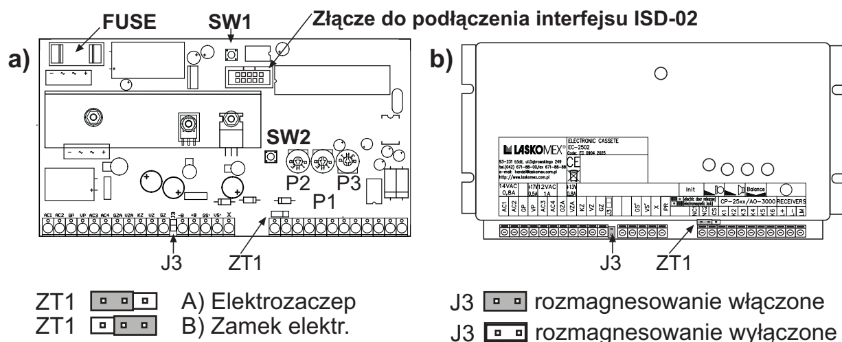
Rysunek 2: Wybór elektrozaczepu lub zamka elektromagnetycznego
