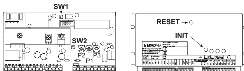
Rysunek 4: Położenie przycisków INIT i RESET
