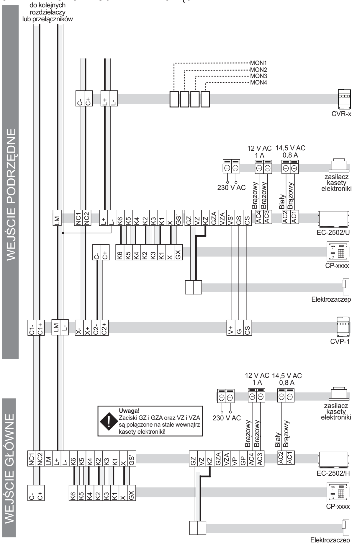
Rysunek 7: Domofon CD-2502 wideo - system wielowejsciowy
