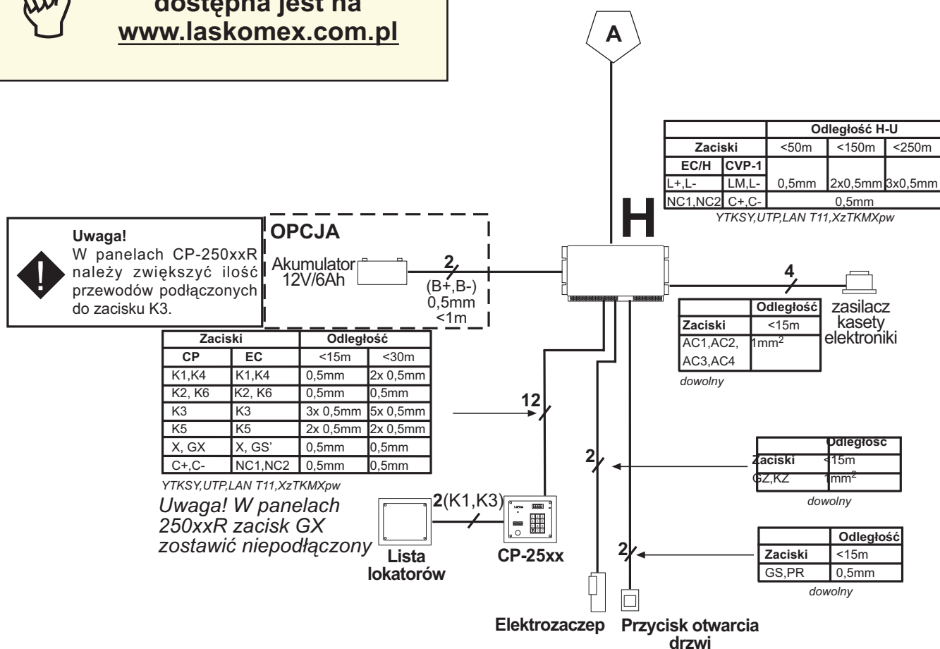
Rysunek 9: Dobór przewodów dla domofonu CD-2502 w wersji wideo - cz.2
