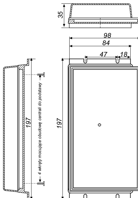
Rys. 13.1 Wymiary kasety elektroniki
