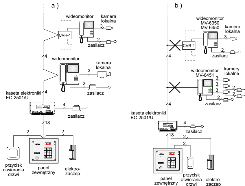
Rys. 7.1 Wykonanie instalacji elektrycznej wideodomofonu: prawidłowa (a) i nieprawidłowa (b)
