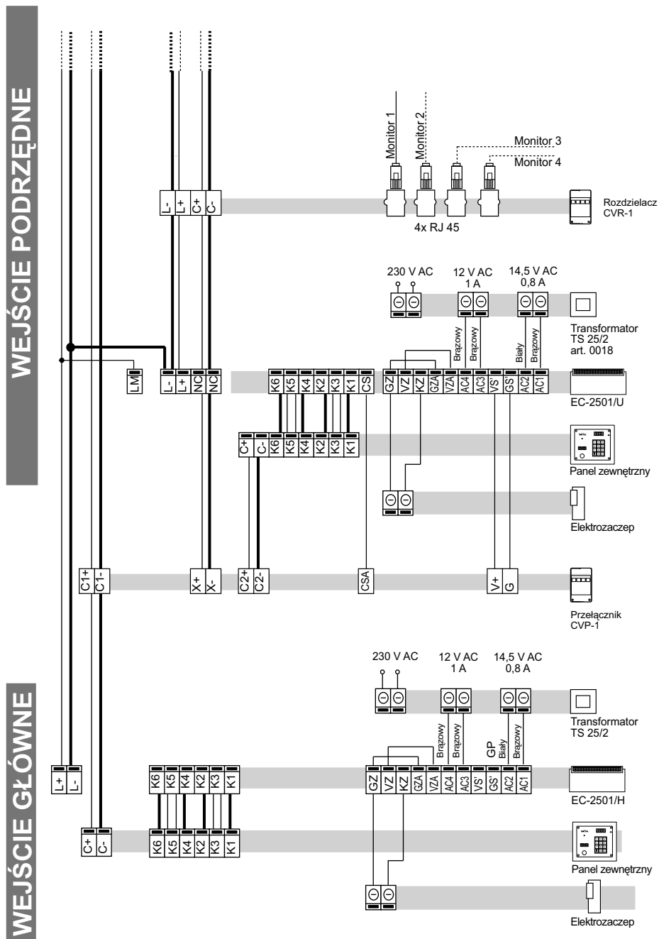
Rys. 13.12 Schemat połączeń systemu wideodomofonowego CD-2501V z wejściem głównym.
