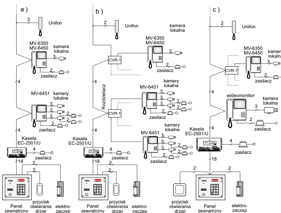
Rys. 6.1 Wideodomofon CD-2501V z wideomonitorami podłączonymi bezpośrednio do magistrali (a), z rozdzielaczami piętrowymi (b), instalacja mieszana (c).
