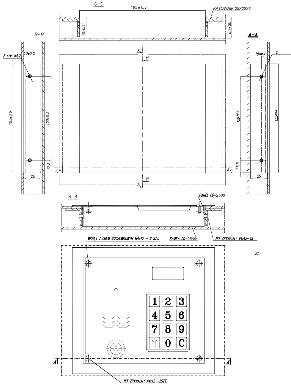
Rys. 13.4 Montaż panela zewnętrznego w nieruchomym skrzydle drzwi od strony przedniej
