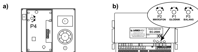
Rys. 7.9 Elementy regulacyjne, a – regulacja wzmocnienie mikrofonu w bramofonie, b –elementy regulacyjne w centrali domofonowej
