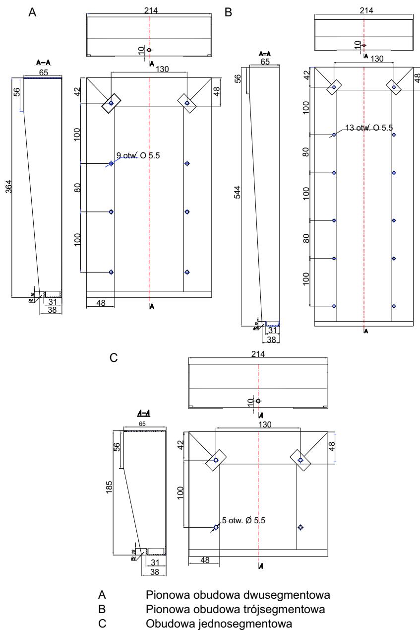
Rys. 13.6 Wymiary obudów natynkowych w układzie pionowym
