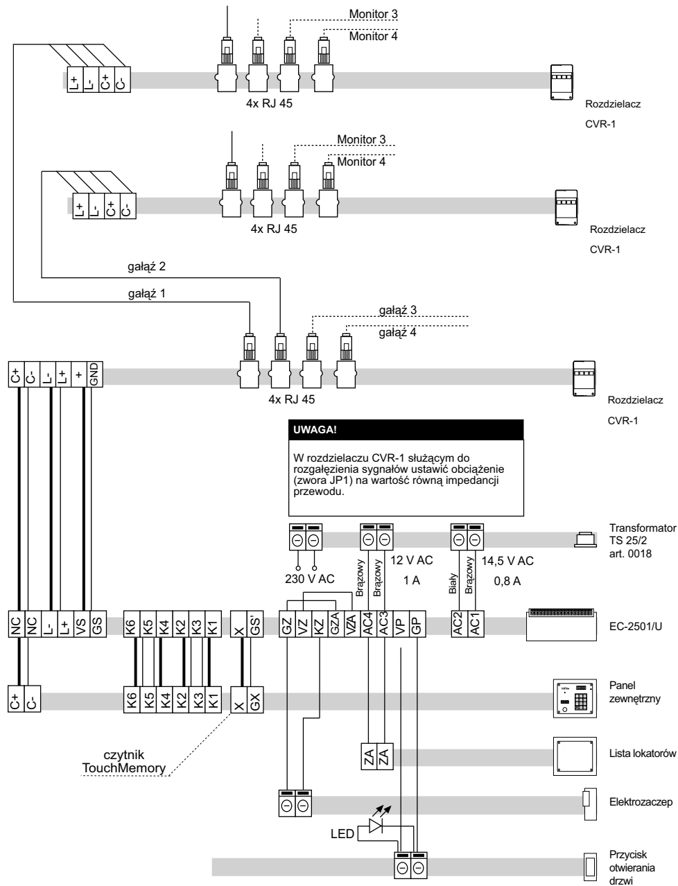
Rys. 13.13 Rozgałęzienie sygnałów w domofonie CD-2501
