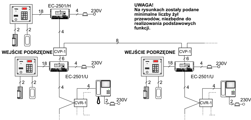
Rys. 6.2 Wiedodomofon w systemie wielowejściowym
