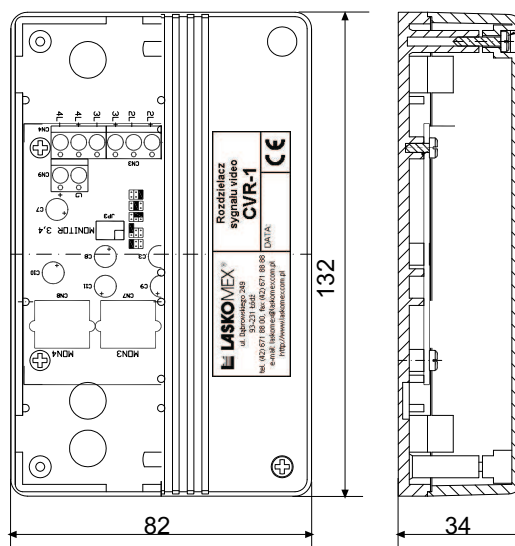
Rys. 13.2 Wymiary rozdzielacza CVR-1
