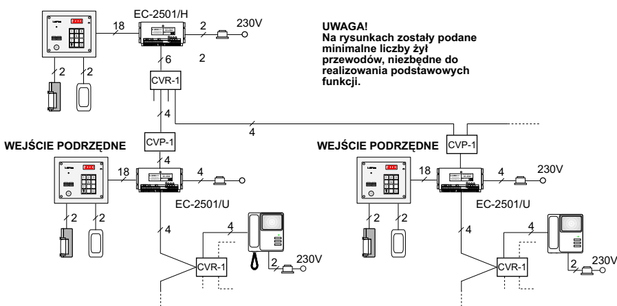
Rys. 6.3 Wiedodomofon w systemie wielowejściowym i przełącznikiem przy wejściu głównym
