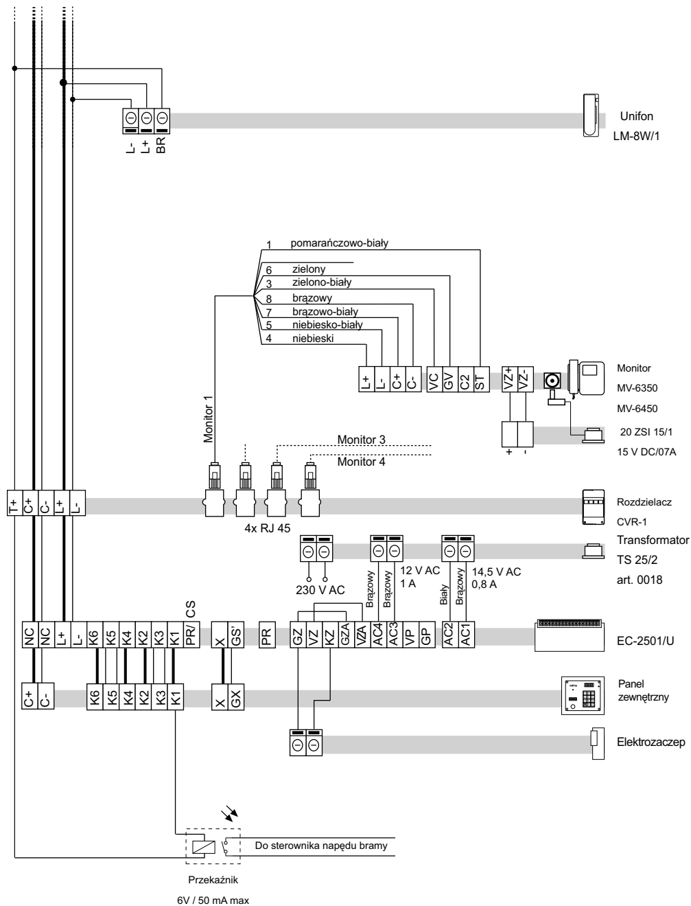
Rys. 13.11 Schemat połączeń systemu CD-2501V z rozdzielaczami sygnału i sterowaniem napędem bramy wjazdowej. Podłączenie akumulatora.
