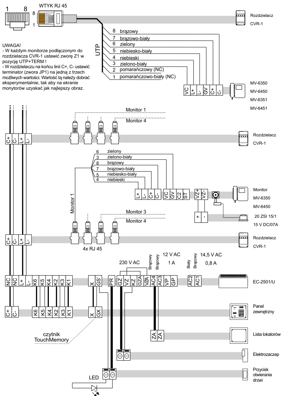
Rys. 13.9 Schemat połączeń systemu wideodomofonowego CD-2501V
