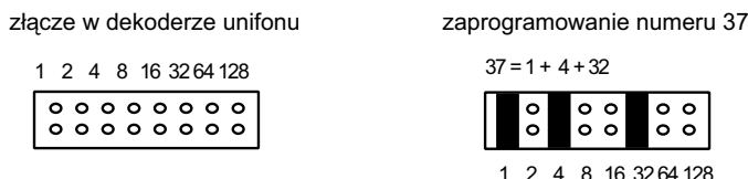
Rys 7.7 Widok złącza służącego do programowania unifonu i przykład ilustrujący zaprogramowanie unifonu na numer 37
