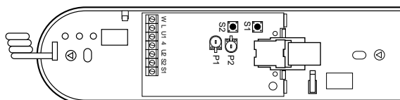
Rys. 3.4 Unifon LM-15.
