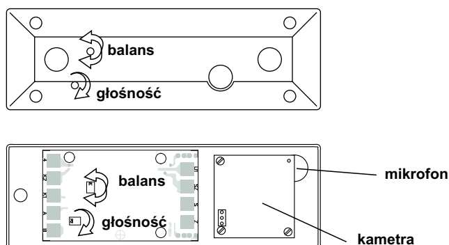
Rys. 6.1 Elementy regulacyjne w bramofonie
