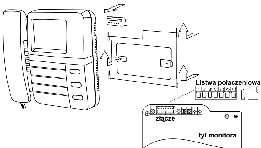
Rys. 5.3 Mocowanie monitora i listwy połączeniowej
