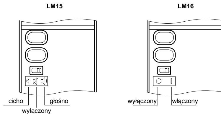
Rys. 7.1 Regulacja głośności wywołania
