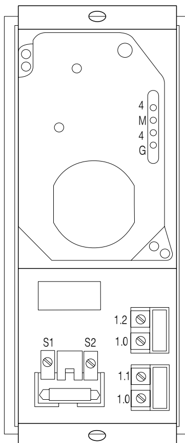
Zaciski panelu rozmównego z dwoma przyciskami (K06502)
