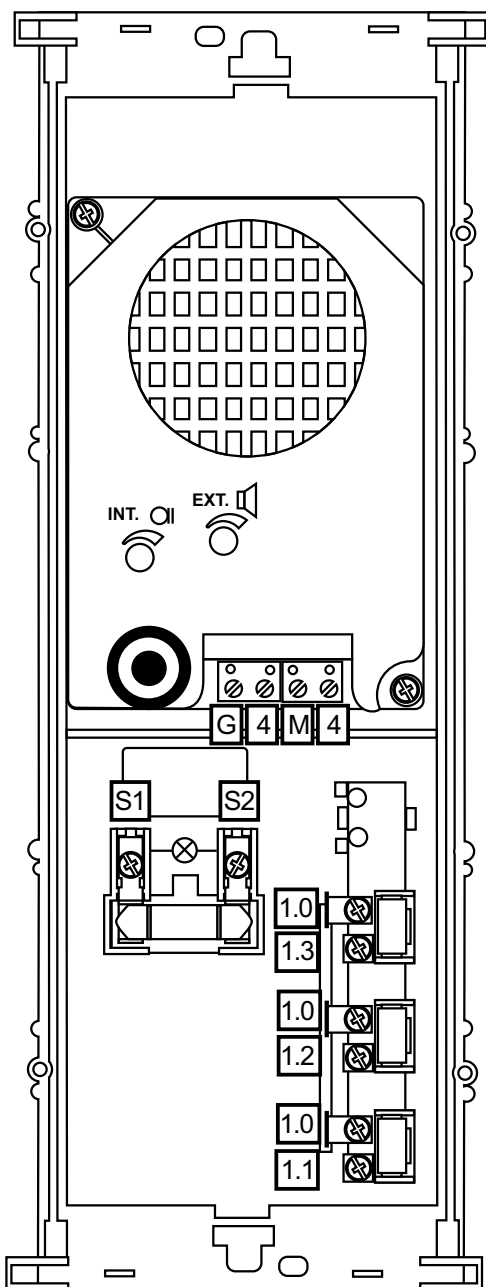
Zaciski panelu rozmównego z trzema przyciskami (725/103)
