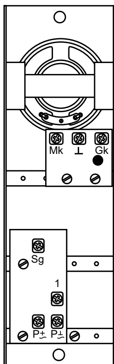
Zaciski panelu rozmównego z jednym przyciskiem (KR-1P)
