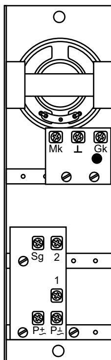
Zaciski panelu rozmównego z dwoma przyciskami (KR-2P)
