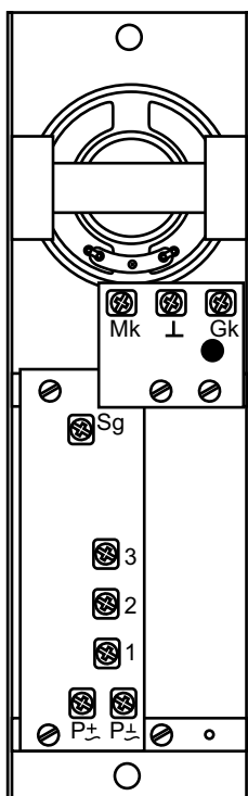
Zaciski panelu rozmównego z trzema przyciskami (KR-3P)
