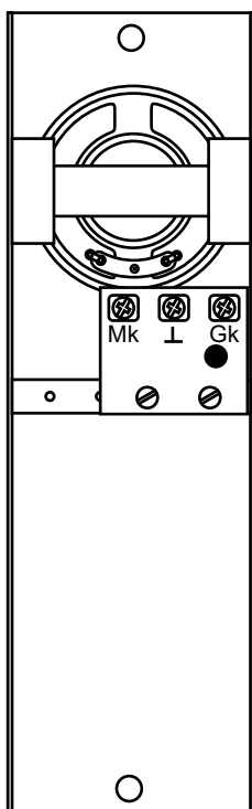
Zaciski panelu rozmównego bez przycisku (KR)
