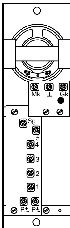
Zaciski panelu rozmównego z pięcioma przyciskami (KR-5P)
