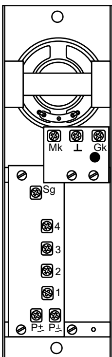
Zaciski panelu rozmównego z czterema przyciskami (KR-4P)
