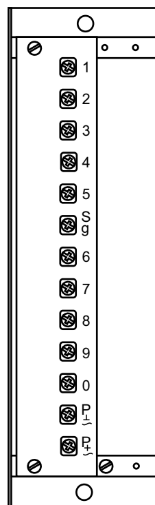
Zaciski panelu numerowego z dziesięcioma przyciskami (K-10P)
