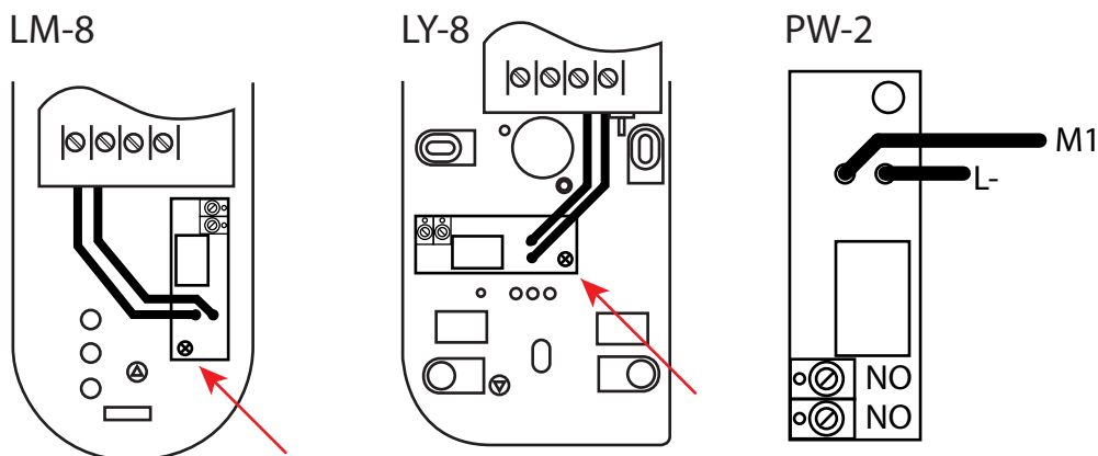
Rys. 2 Montaż modułu PW-2 w unifonach w unifonach LY-8 i LM-8
