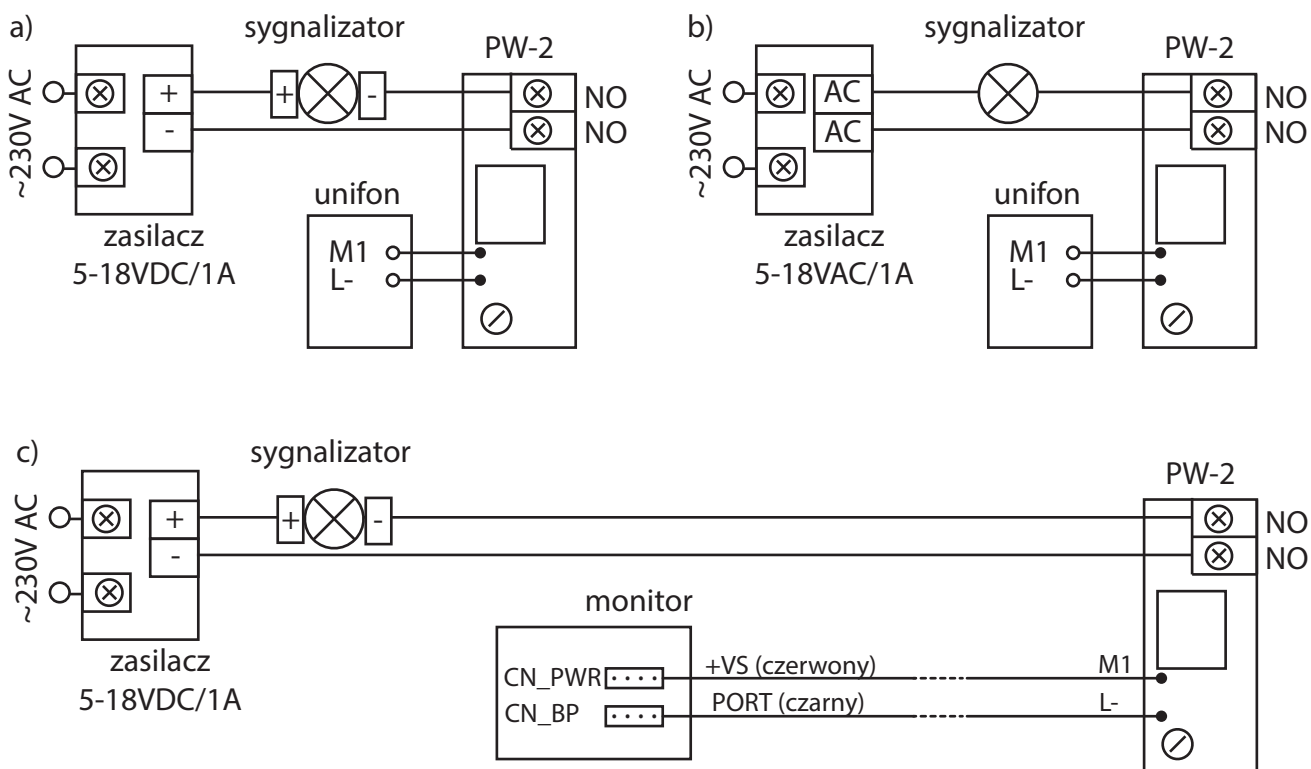
Rys. 2 Montaż modułu PW-2 w unifonach w unifonach LY-8 i LM-8
