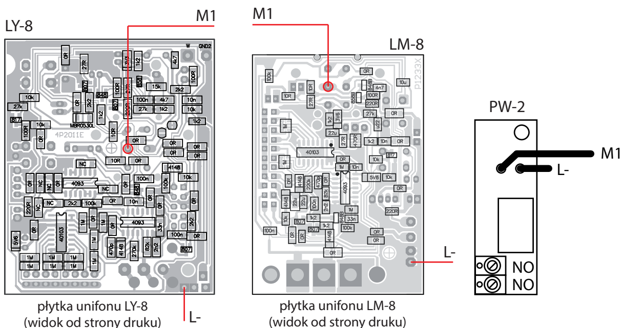
Rys. 1 Podłączenie modułu PW-2 do płytek w unifonach LY-8 i LM-8
