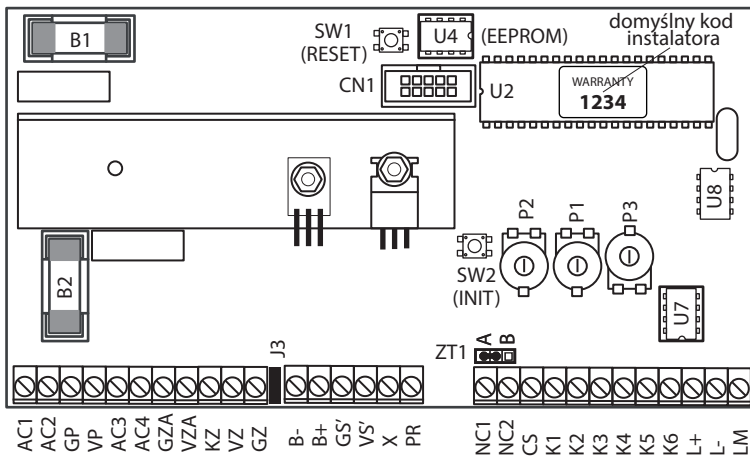
Rys. 13.1 Zaciski centrali domofonowej EC-2502
