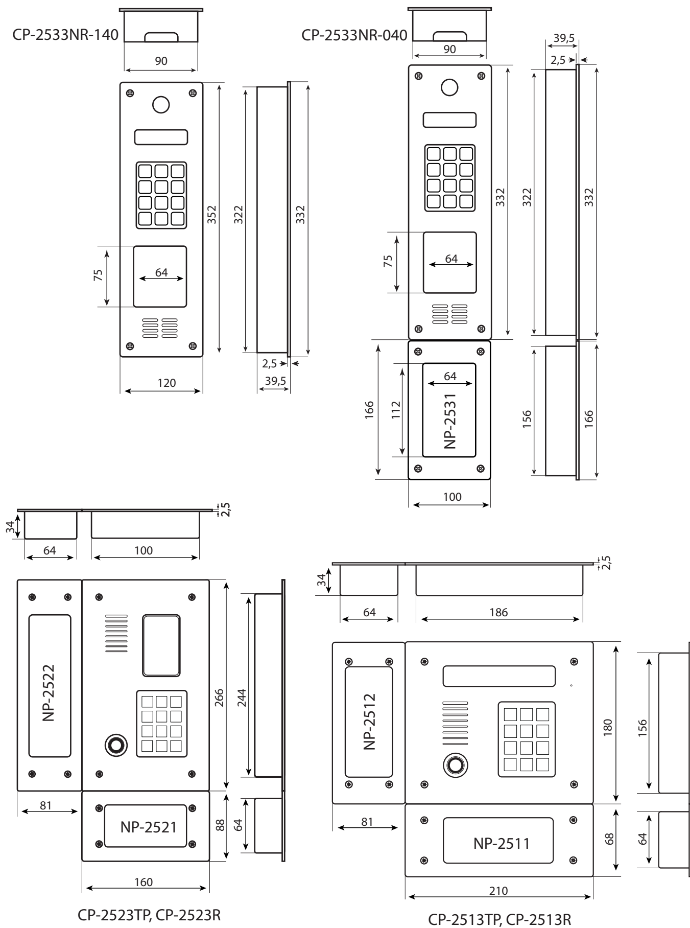
Rys. 13.8 Wymiary paneli zewnętrznych ze stali nierdzewnej INOX
