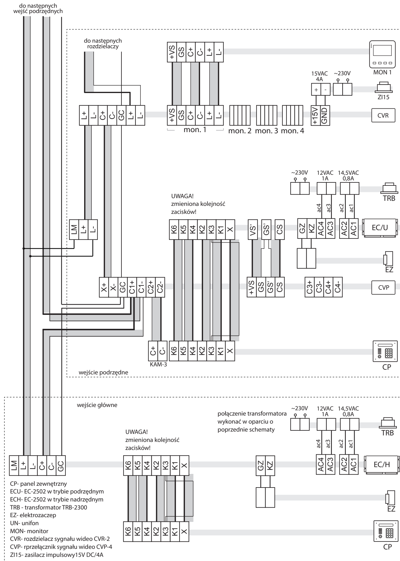
Rys. 14.8 System wideo z wejściem głównym.
