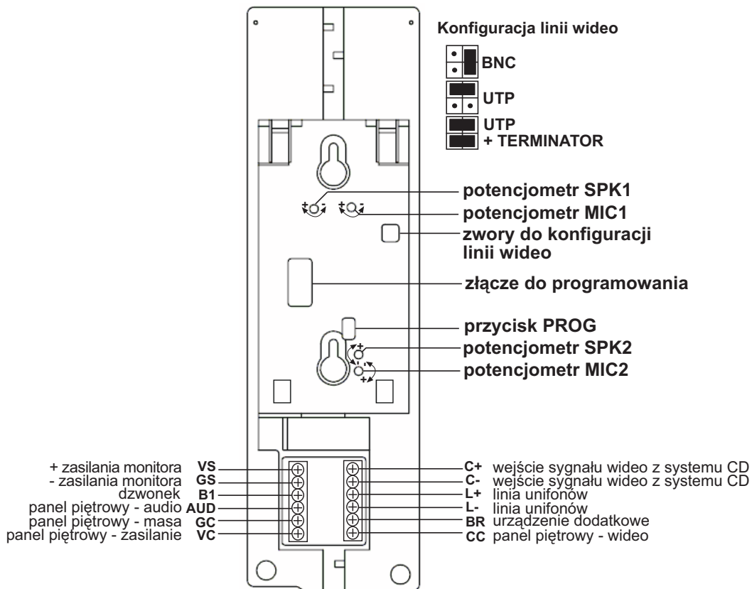
Rys. 2 Widok monitora MVC-6850 z tyłu
