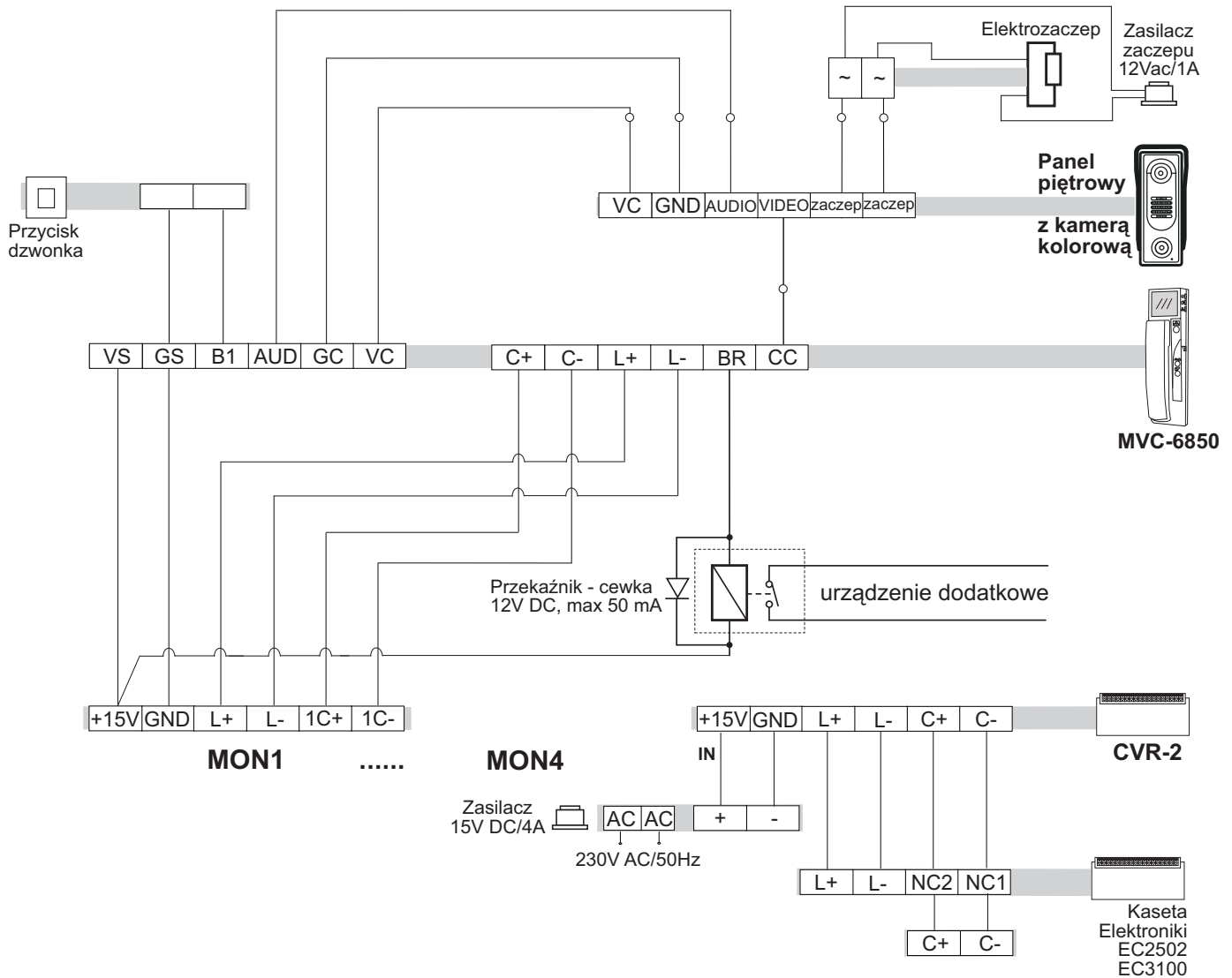
Rys. 4 Schemat połączeń - zasilanie centralne dla 4 monitorów
