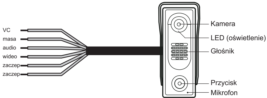
Rys 3. Przykładowy panel piętrowy z kamerą kolorową typu Commax
