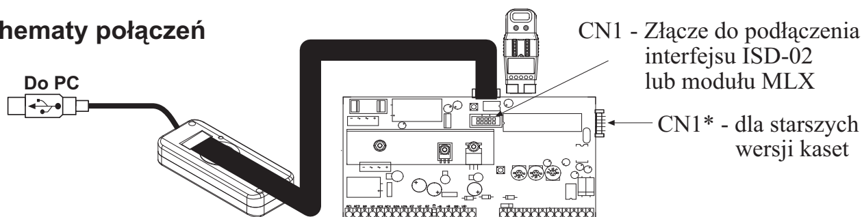
Rys 3. Bezpośrednie połączenie kasyety EC z interfejsem ISD-02 lub modułem MLX
