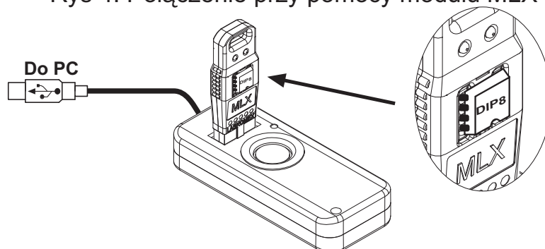
Rys 5. Odczyt/zapis z/do pamięci DIP wyjętej z centrali EC i włożonej do modułu MLX
