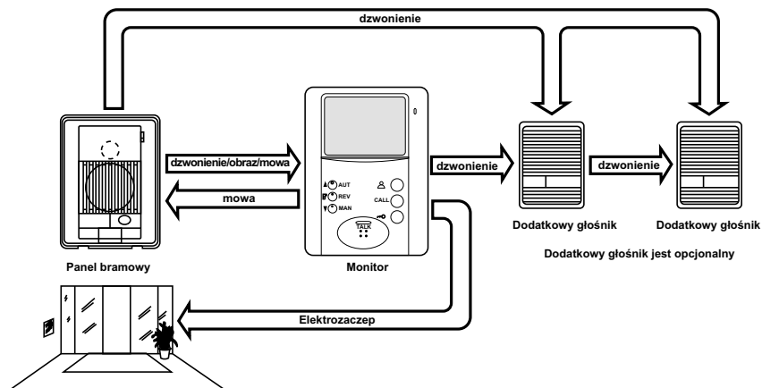
Zasada działania wideodomofonu Telecall
