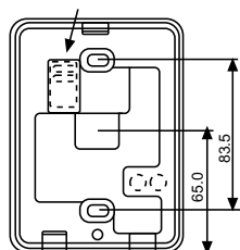
Tył panela
