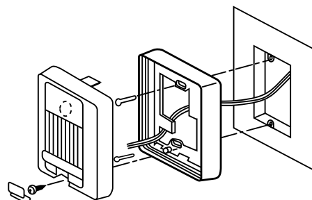
Montaż kasety rozmównej
