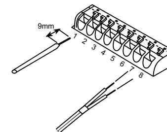
Złącze do podłączenia przewodów
