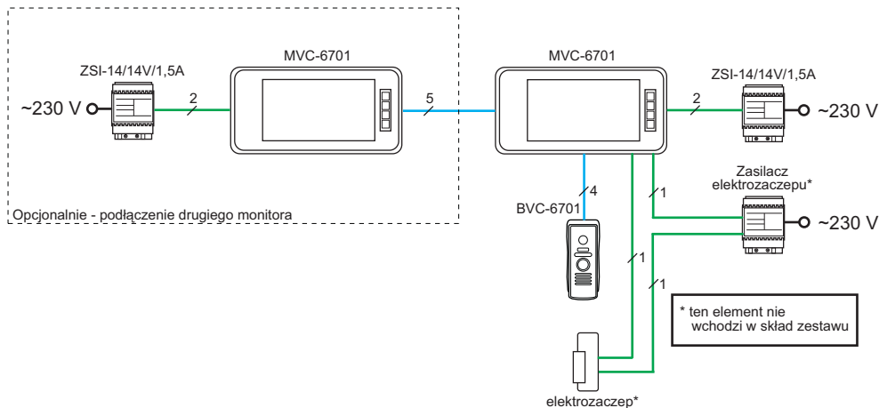
Rys 5. Podłączenie zestawu widetelny Taurus - schemat jednokreskowy
