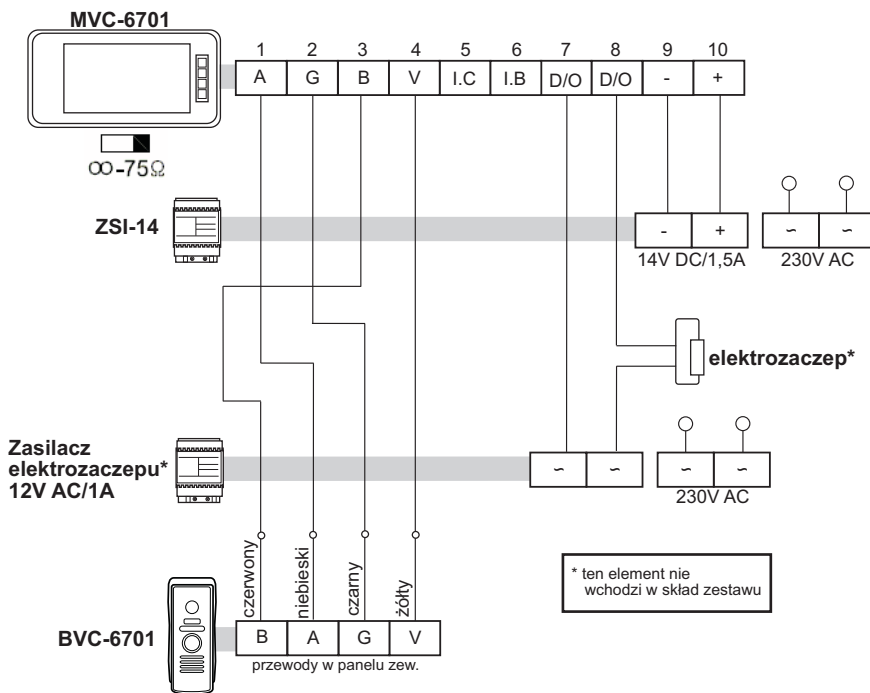
Rys 6. Schemat ideowy podłączenia elementów zestawu widetelny Taurus
