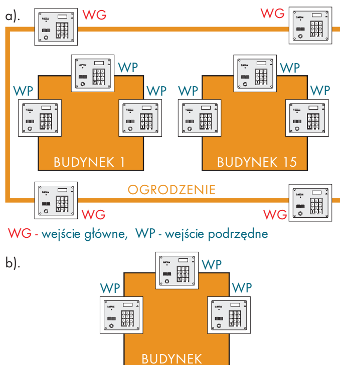
Rys. 1 Przykładowe zastosowanie domofonu CD-3100 w ogrodzonej grupie budynków a) klatce schodowej z trzema wejściami b).
