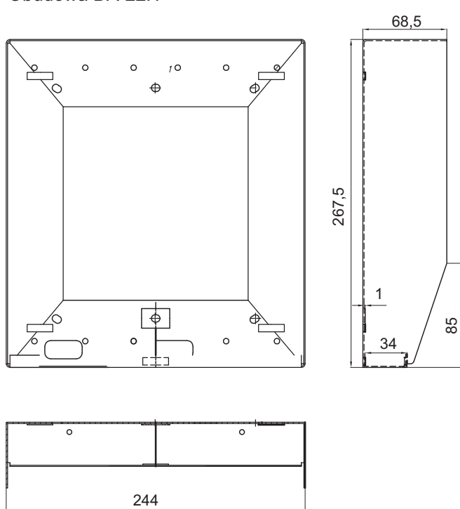
Obudowa DA-22H
