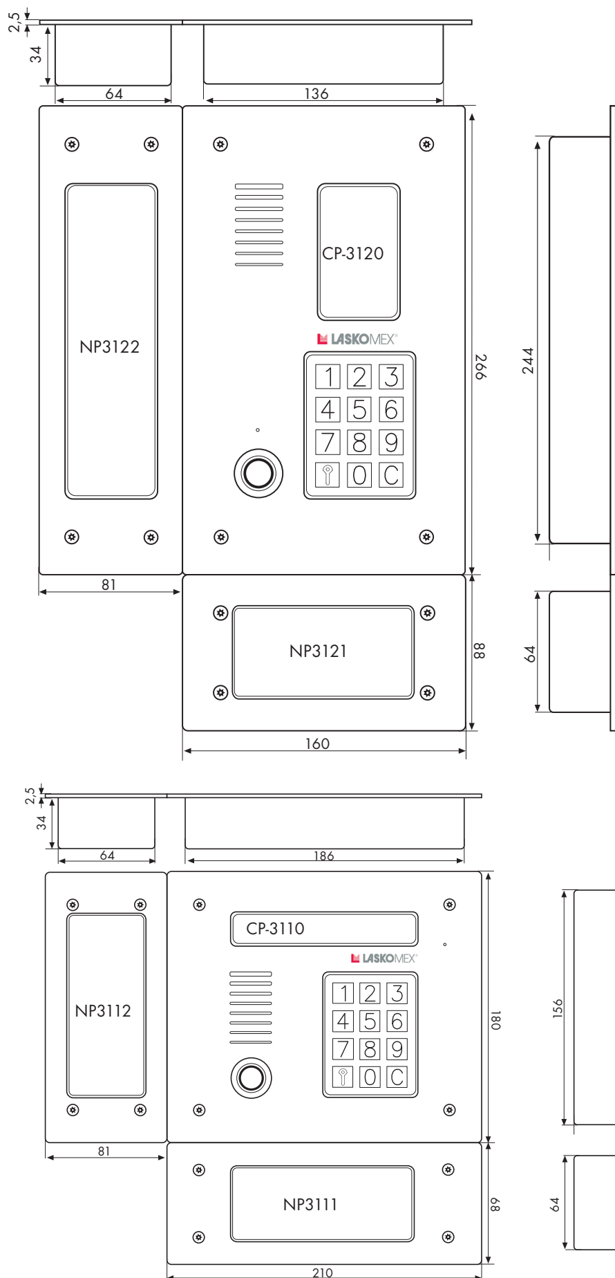
Rysunek 7. Wymiary paneli ze stali nierdzewnej (Inox)
