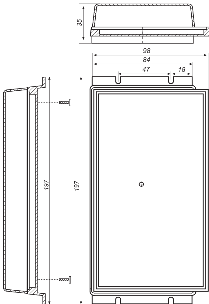
Rysunek 9. Wymiary kasety elektroniki
