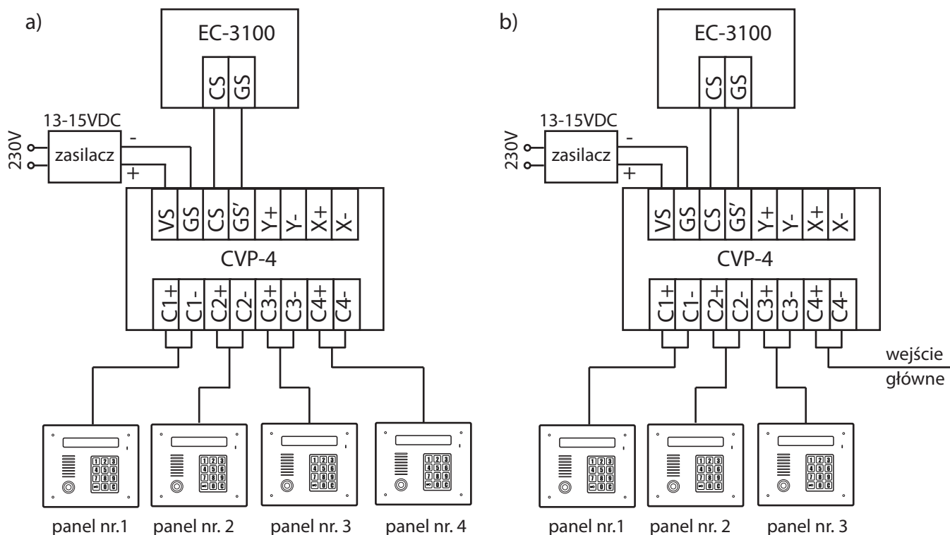
Rys.2 Przełącznik CVP-4 w systemie CD-3100 przy wejściu głównym a) i przy wejściu podrzędnym b)
