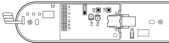
Rys. 3.4 Unifon LM-15/1.
